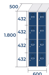
ECOC-30/2 PRO 38,6kg . 0,54m 3
