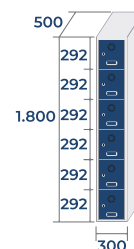
ECOB-30/1 PRO 24,5kg . 0,27m 3
