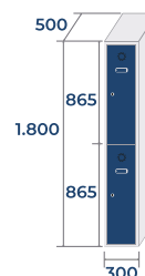
ECOT-30/1 PRO 19,1kg · 0,27m 3
