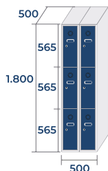
ECOM-25/2 PRO 33,8kg . 0,45m 3
