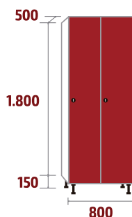
FV-40/2 84,85kg . 0,71m 3
