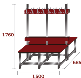
BANC-2-1500-FEN-INOX 64kg · 0,6m 3 · 16 ↓
