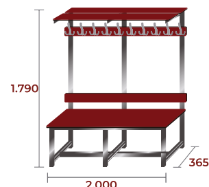
BANC-3-2000-FEN-INOX 43,5kg · 0,31m 3 · 10 ↓
