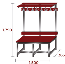
BANC-3-1500-FEN-INOX 38,5kg · 0,3m 3 · 8 ↓
