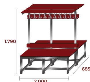
BANC-3-2000-FEN-INOX 87kg · 0,62m 3 · 20 ↓
