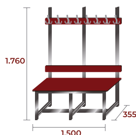
BANC-2-1500-FEN-INOX 32kg · 0,3m 3 · 8 ↓
