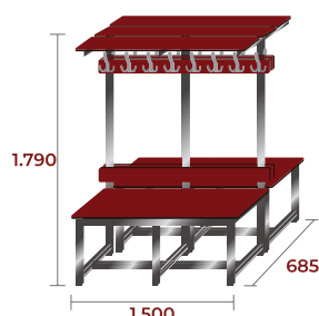
BANC-3-1500-FEN-INOX 77kg · 0,6m 3 · 16 ↓
